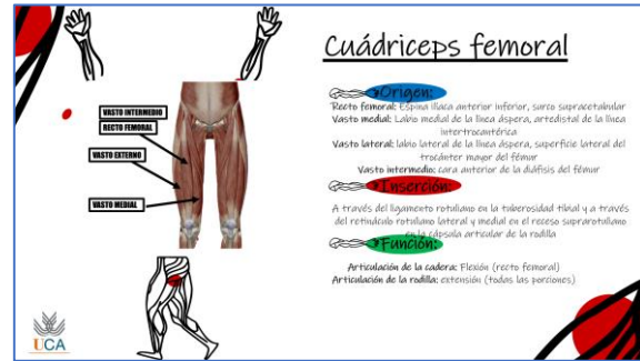
Imagen 1: Diseño de la flashcard realizada por los propios alumnos del curso de Anatomía humana del Grado de Ciencias de la Actividad Física y Deporte.
